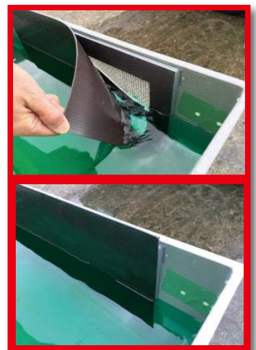
浸水時(止水シート取り付け)
